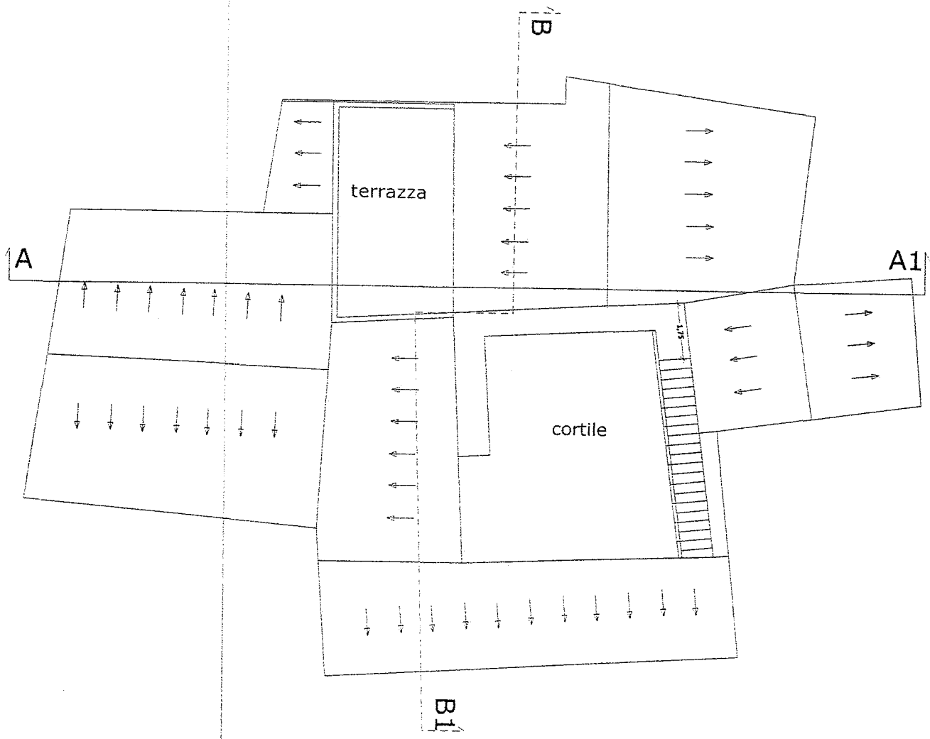
PIANTA DELLE COPERTURE
