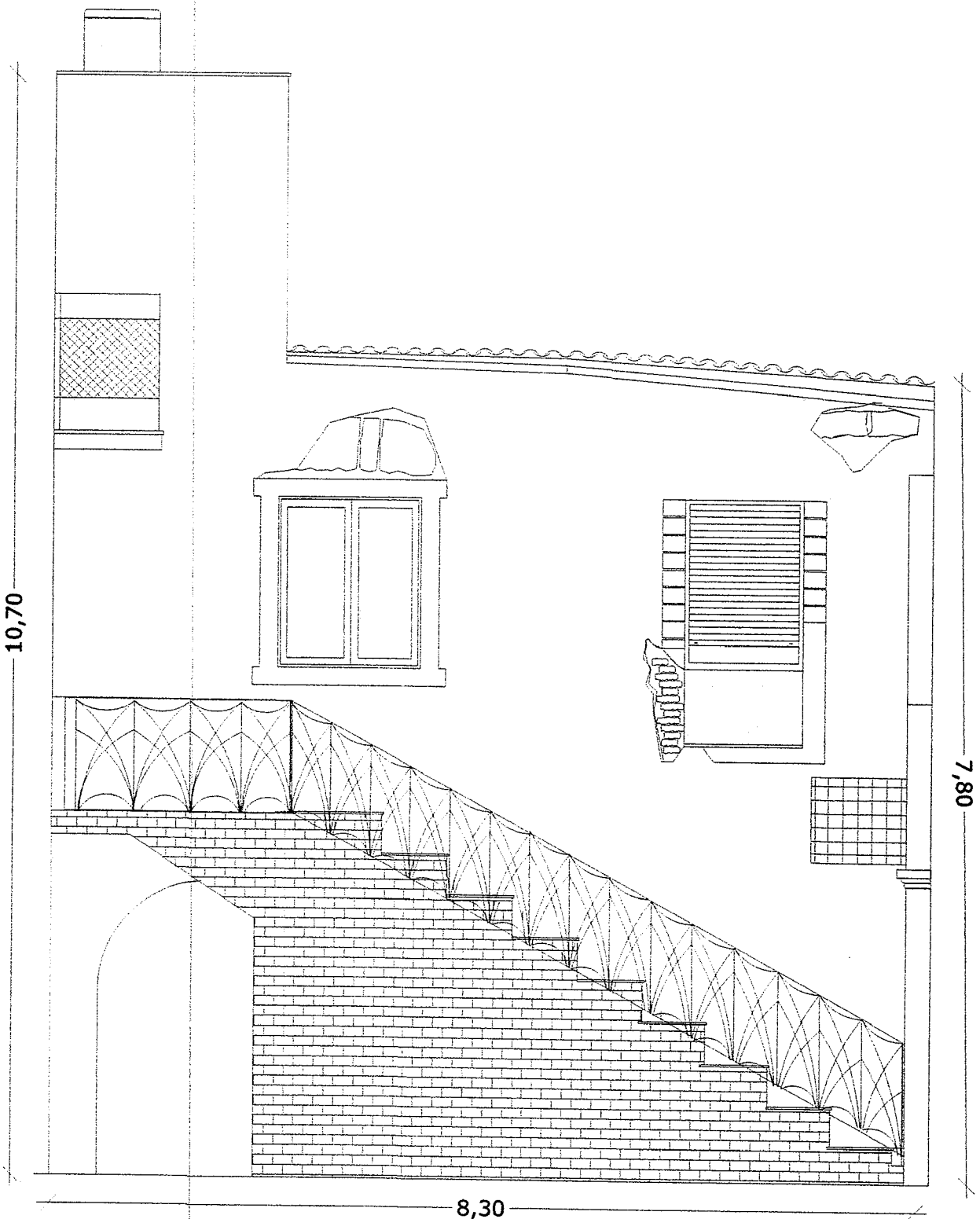
prospetto nord interno
