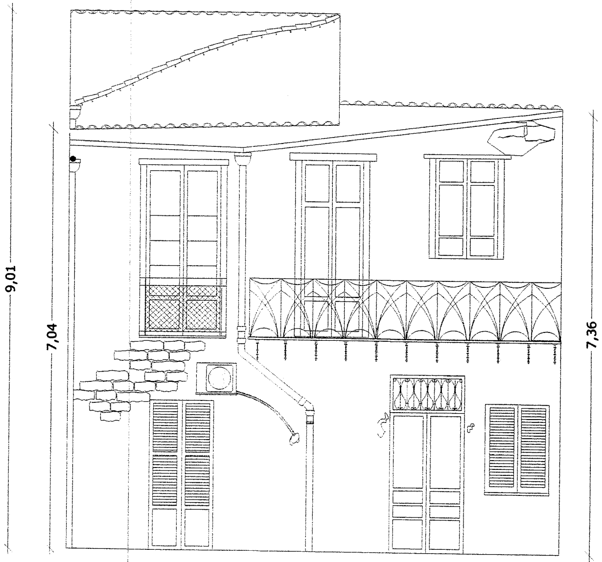
prospetto 8,14 sud interno
